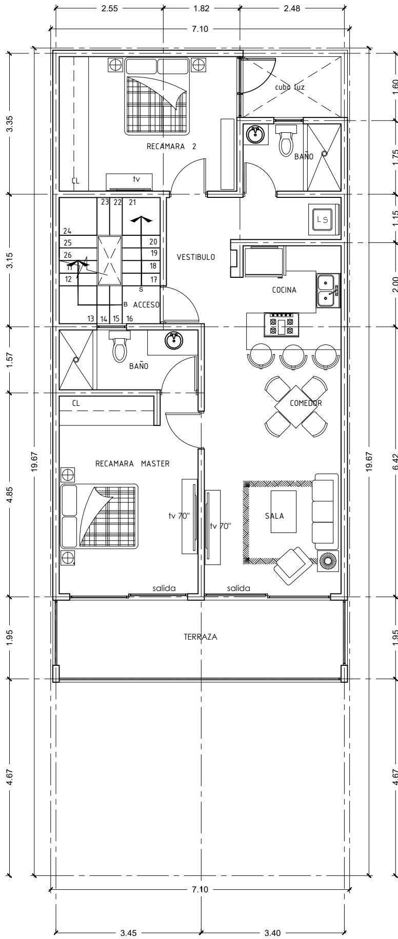
PLANTA ARQ. ALTA TIPO N(+).2.85, N(+).5.70npt
